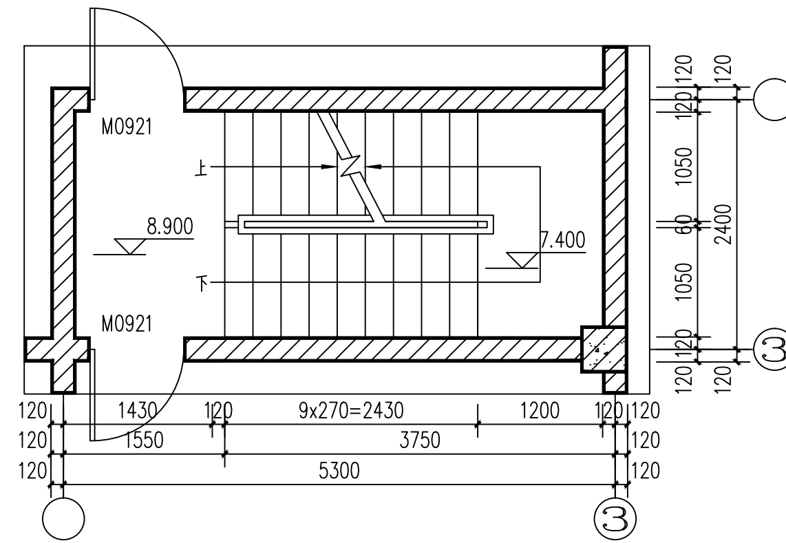
2#三层楼梯平面大样图 1:50
