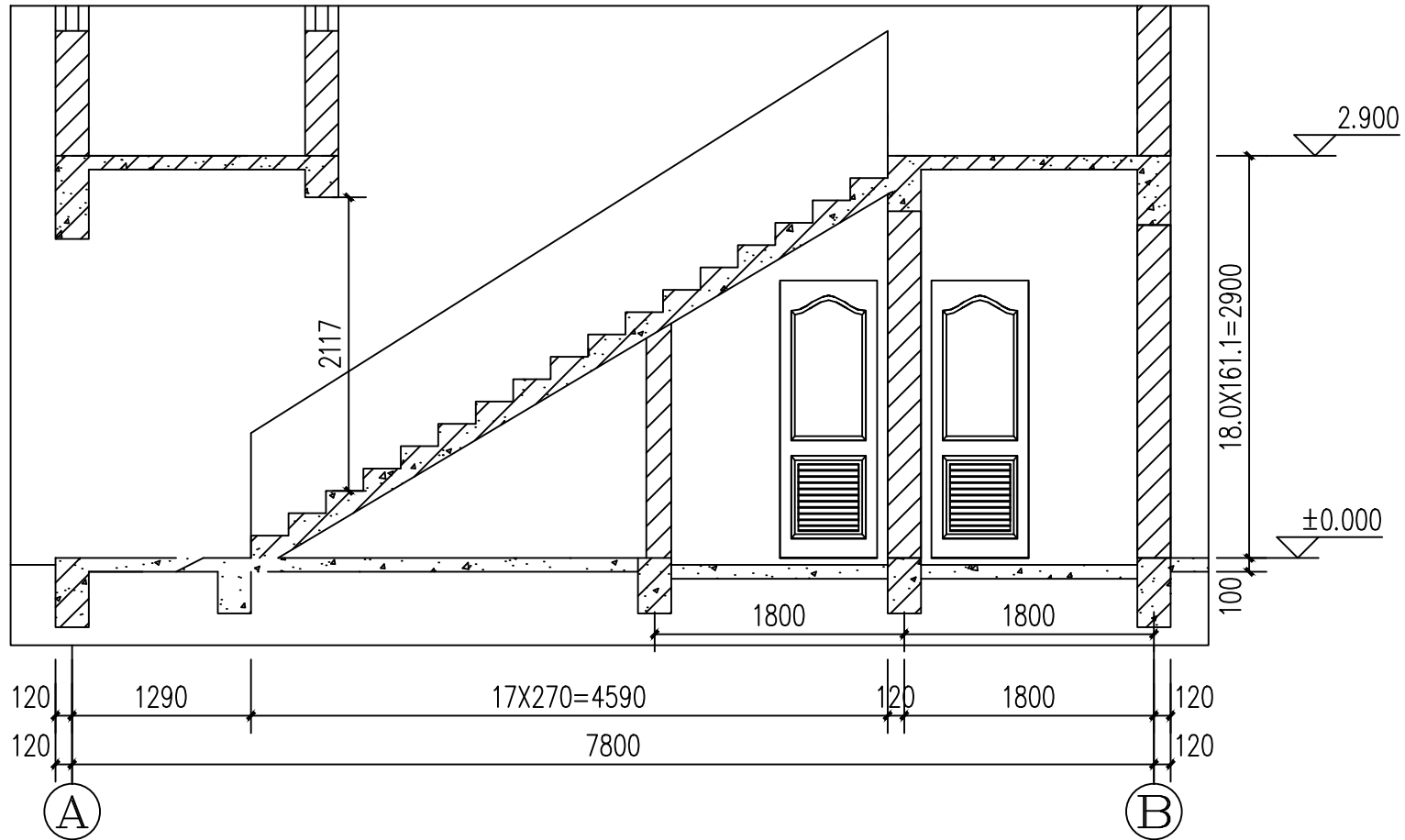
1#楼梯剖面大样图 1:50
