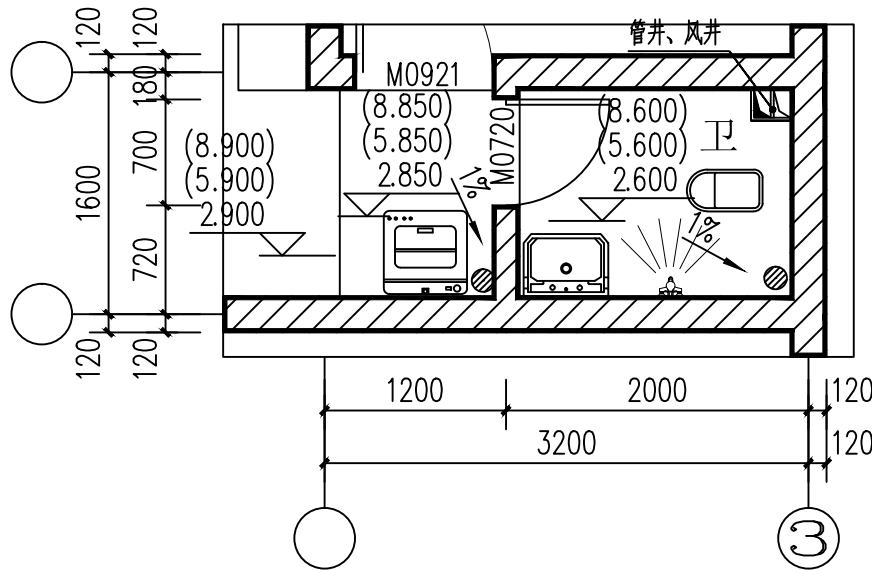
2#卫生间大样 1:50
