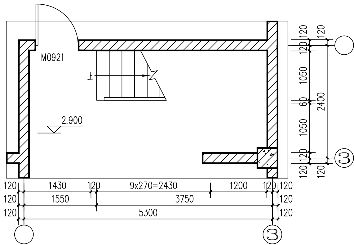
2#一层楼梯平面大样图 1:50
