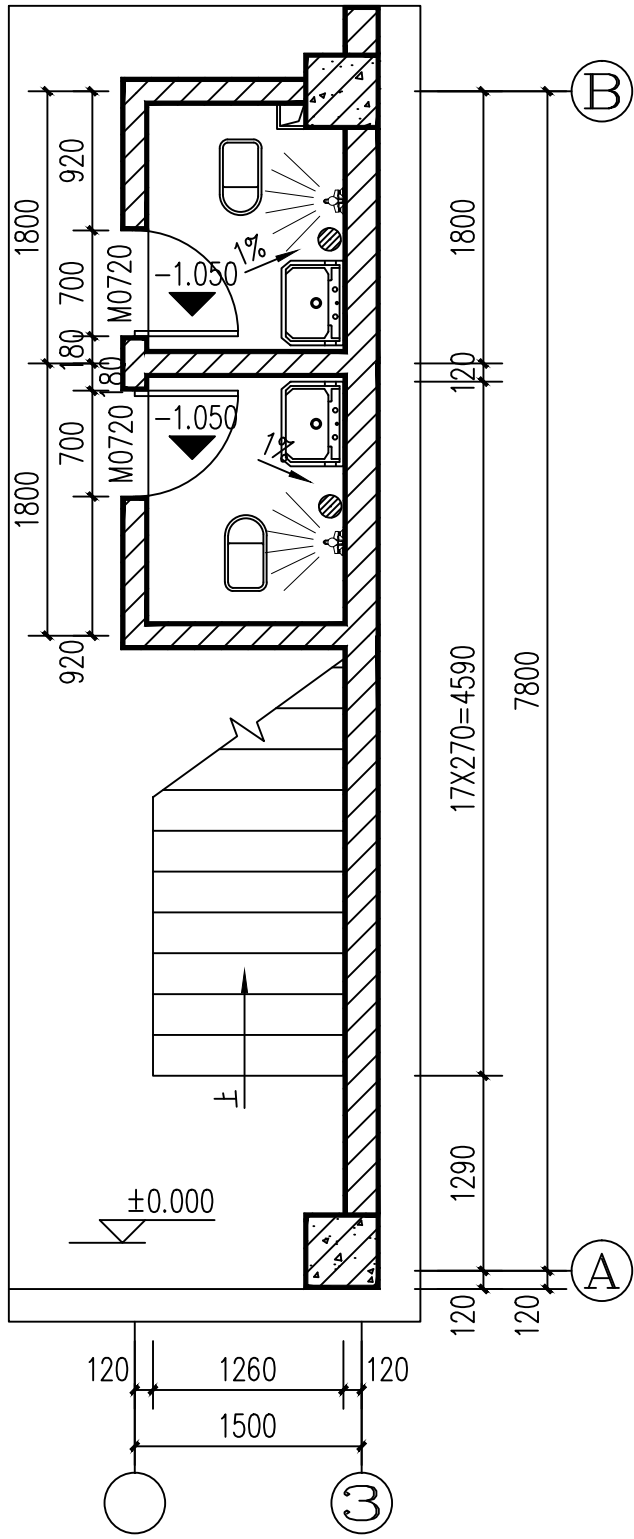
1#一层楼梯平面大样图 1:50
