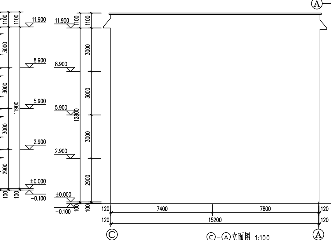
C-A立面图 1:100
