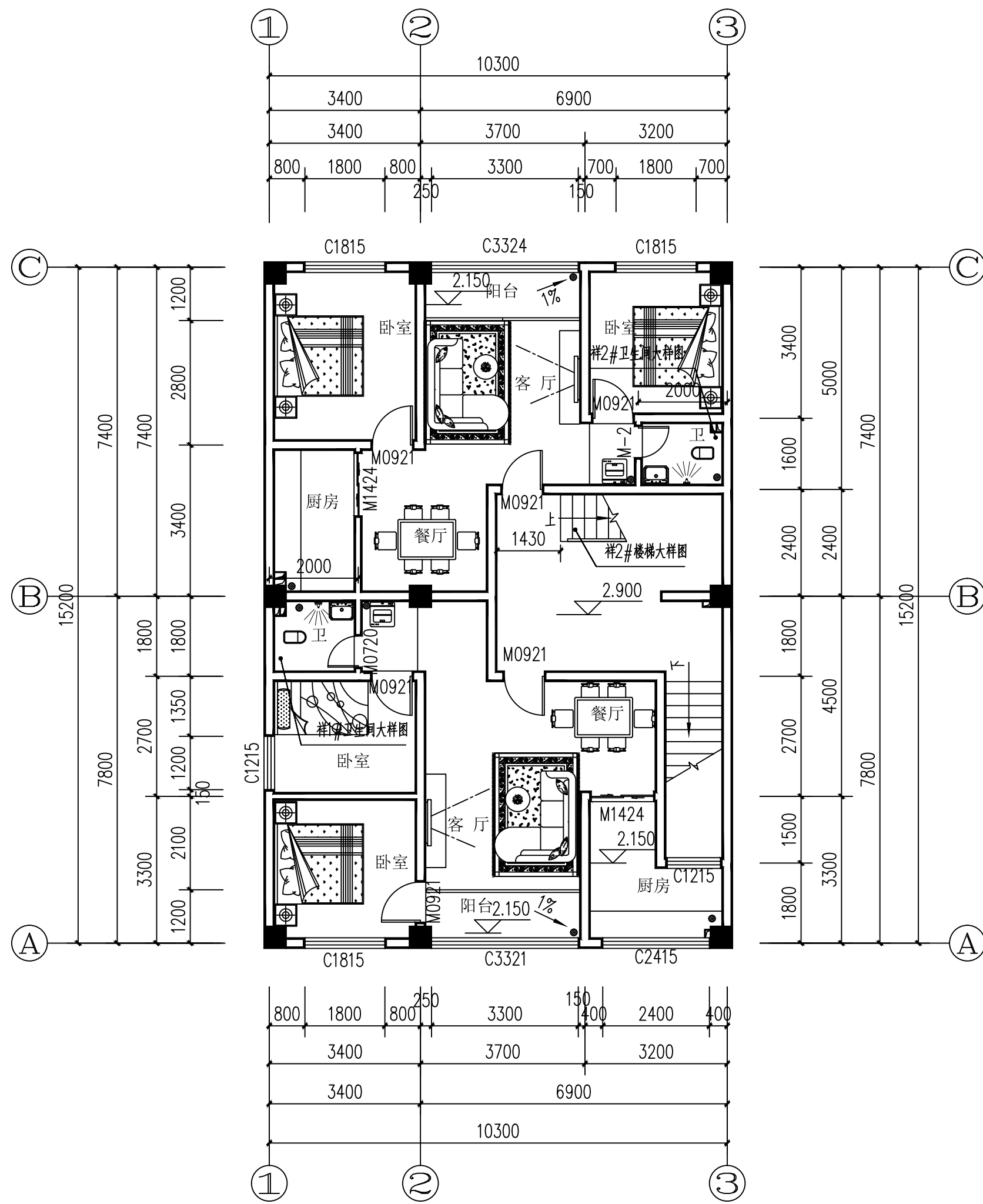
二层平面图
