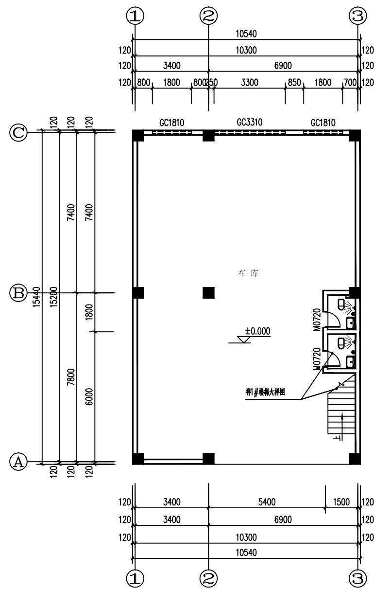
一层平面图 1: 100
