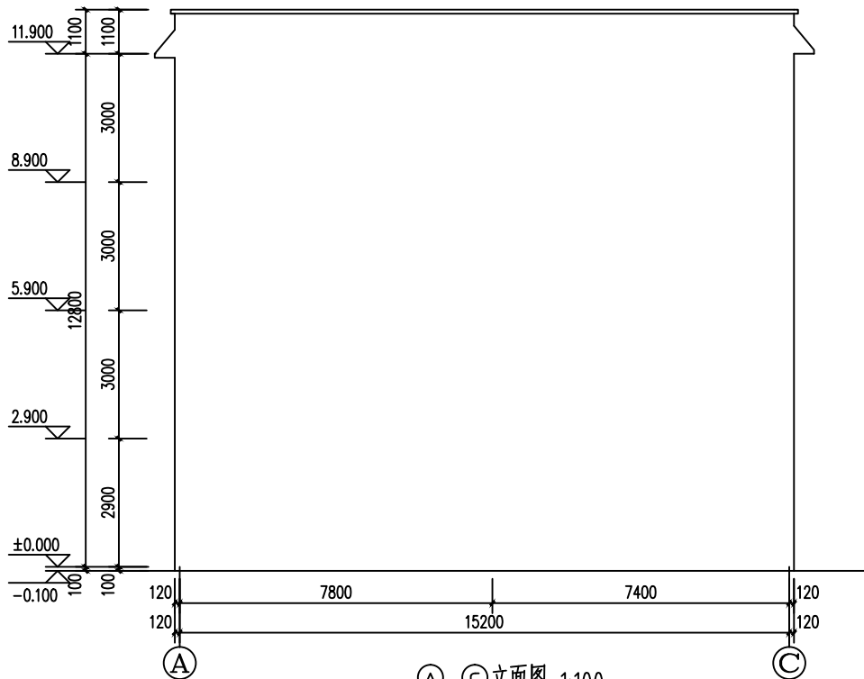
A-C立面图 1:100
