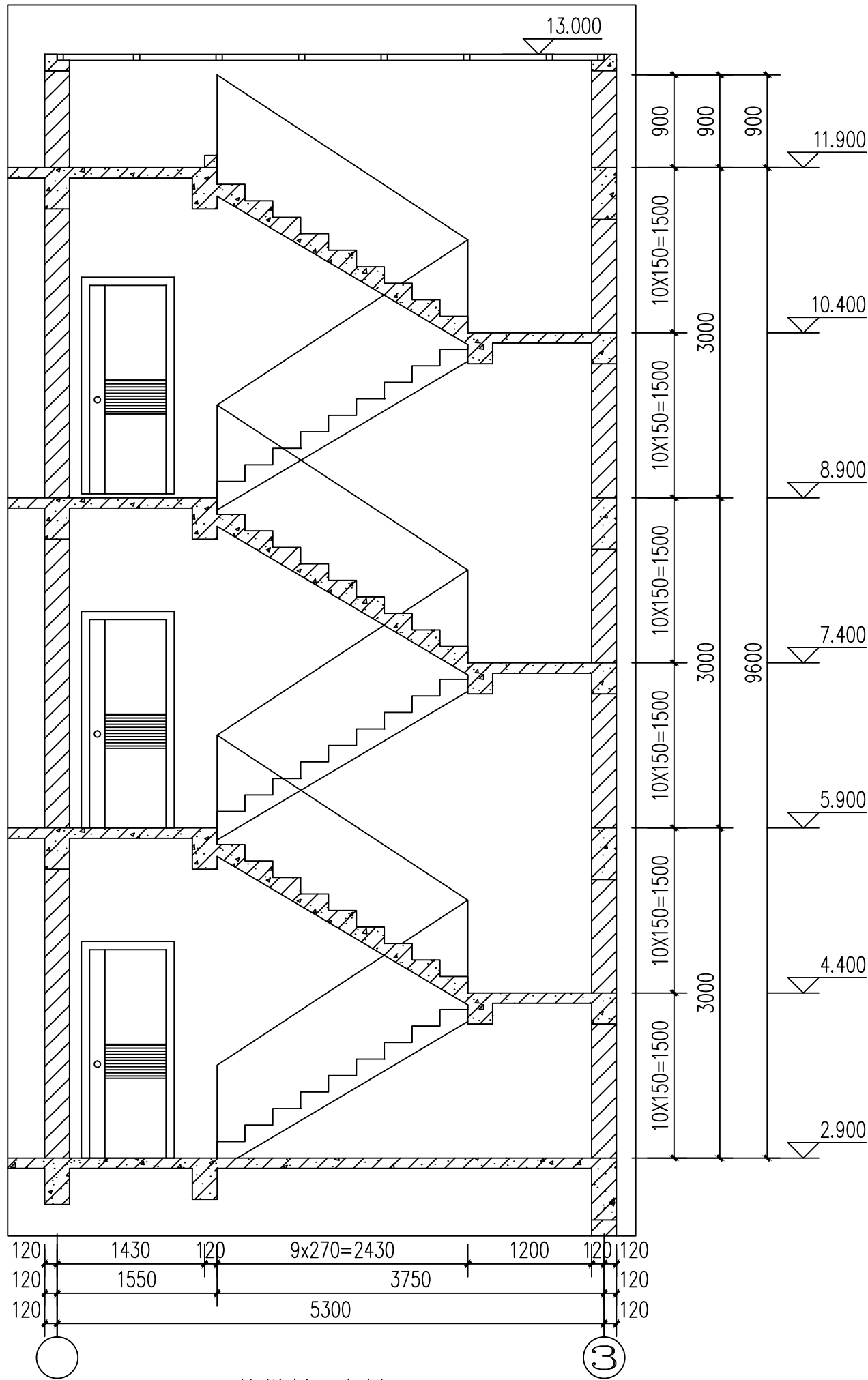
2#楼梯剖面大样图 1:50
