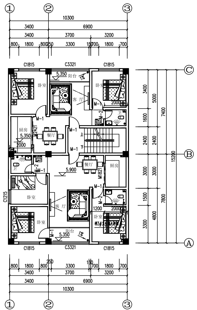
三层平面图 1: 100
