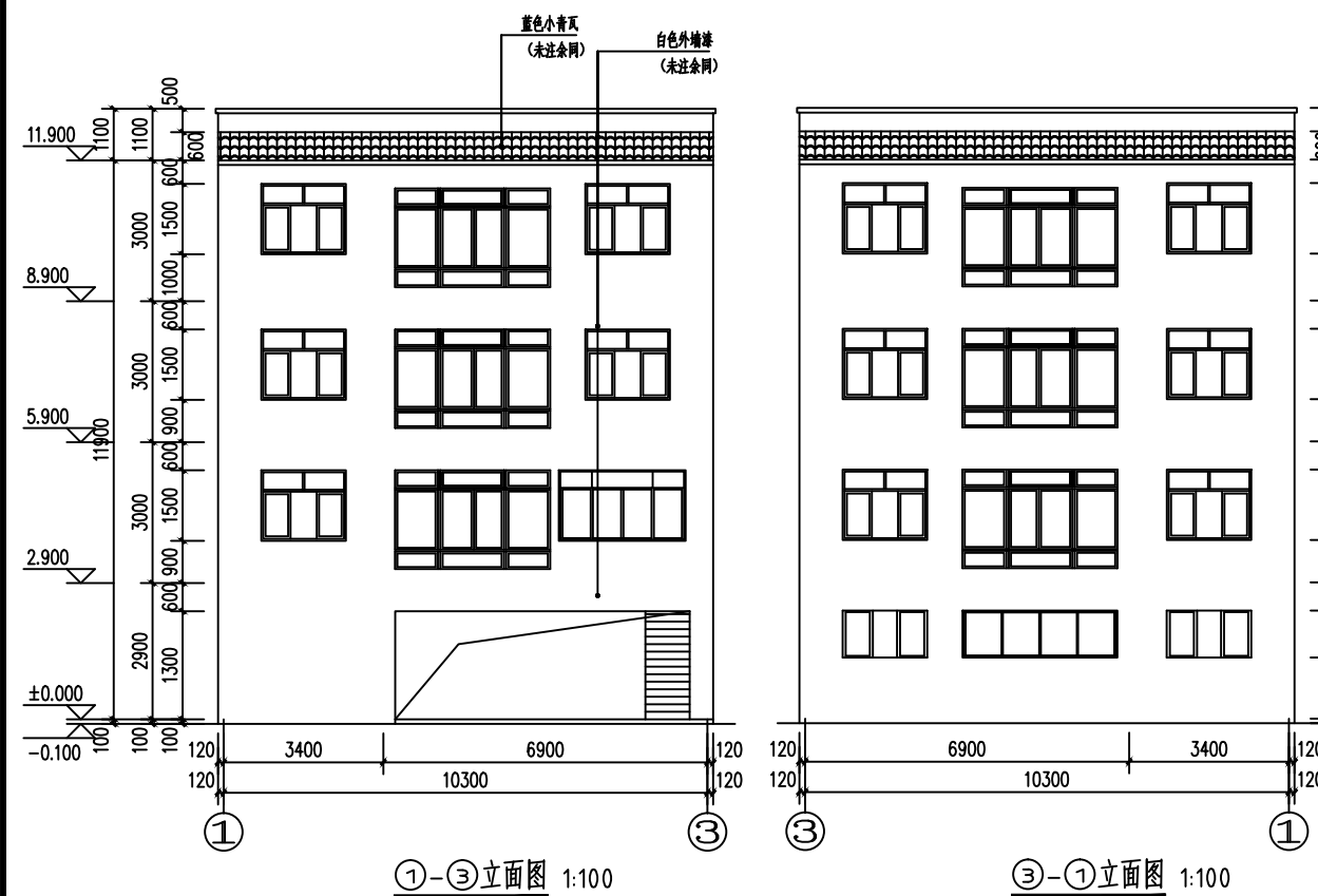
①-③立面图 1:100
