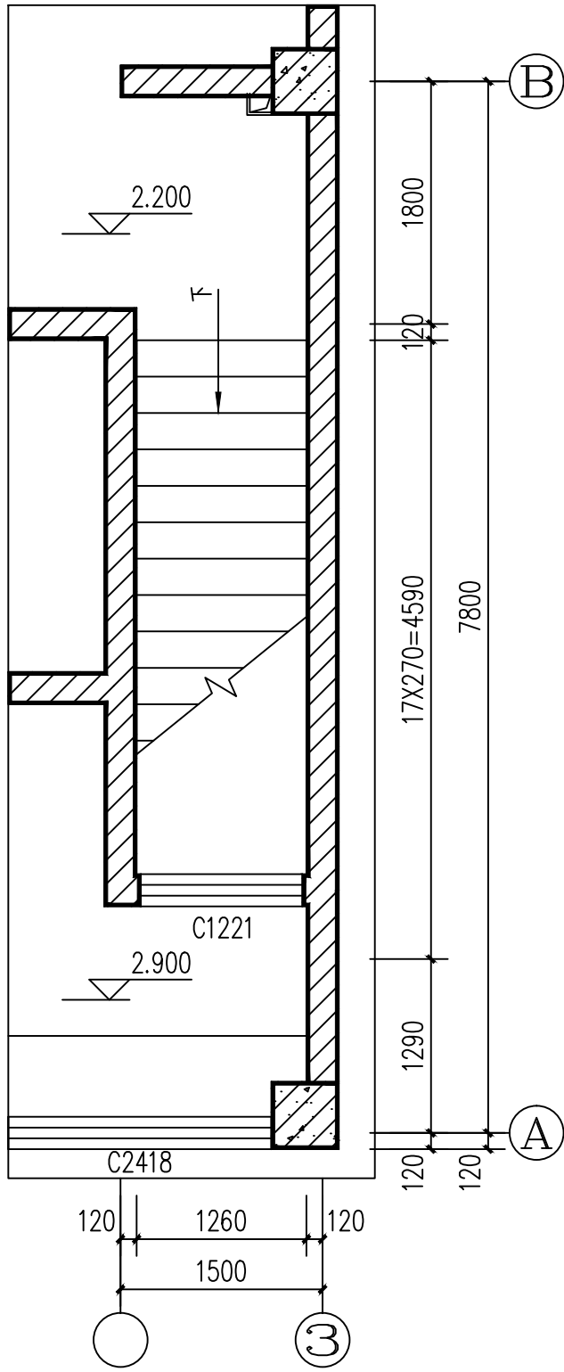
1#二层楼梯平面大样图 1:50
