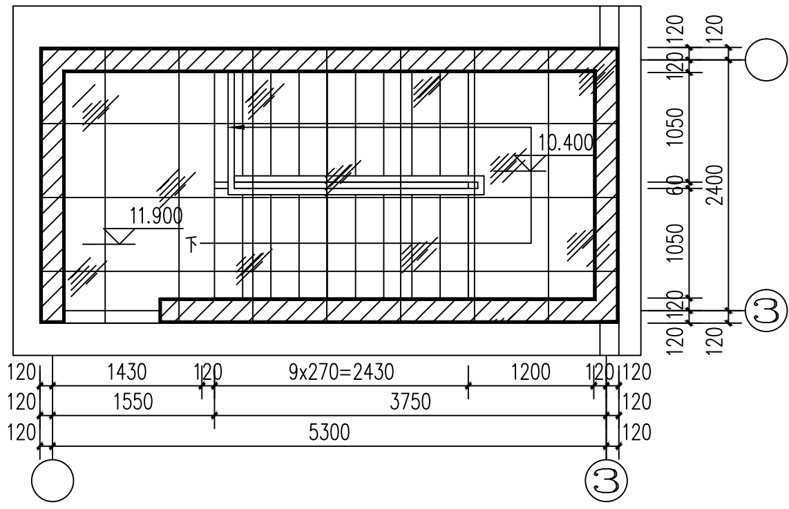
2#屋顶楼梯平面大样图 1:50
