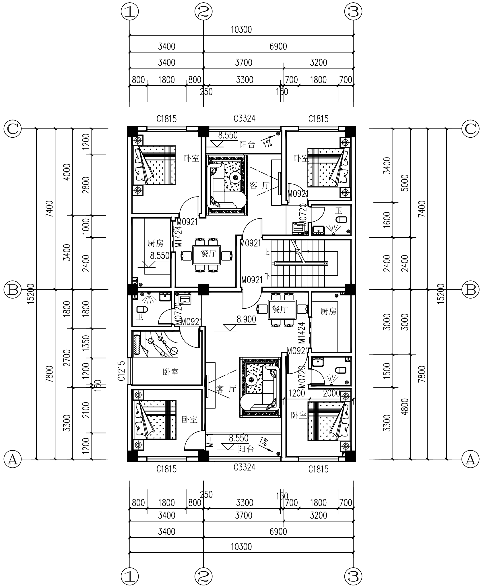
四层平面图 1: 100 四层建筑面积: 162.70m²
