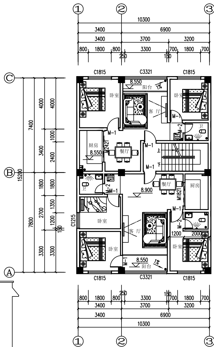
四层平面图 1: 100
