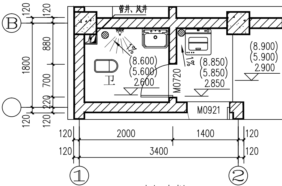
1#卫生间大样 1:50
