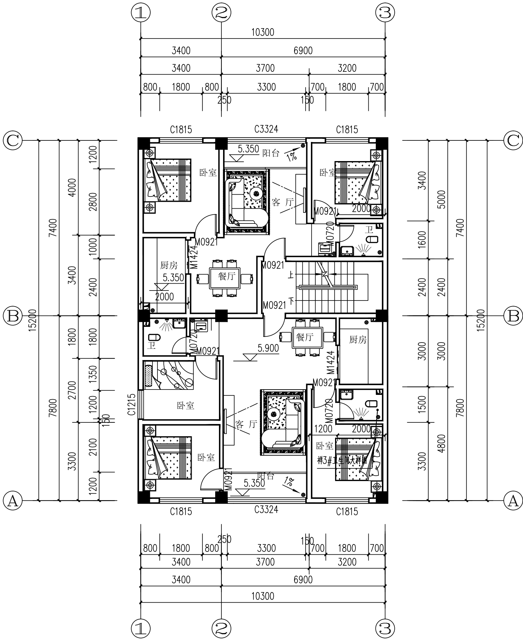
三层平面图 1: 100 三层建筑面积: 162.70m²
