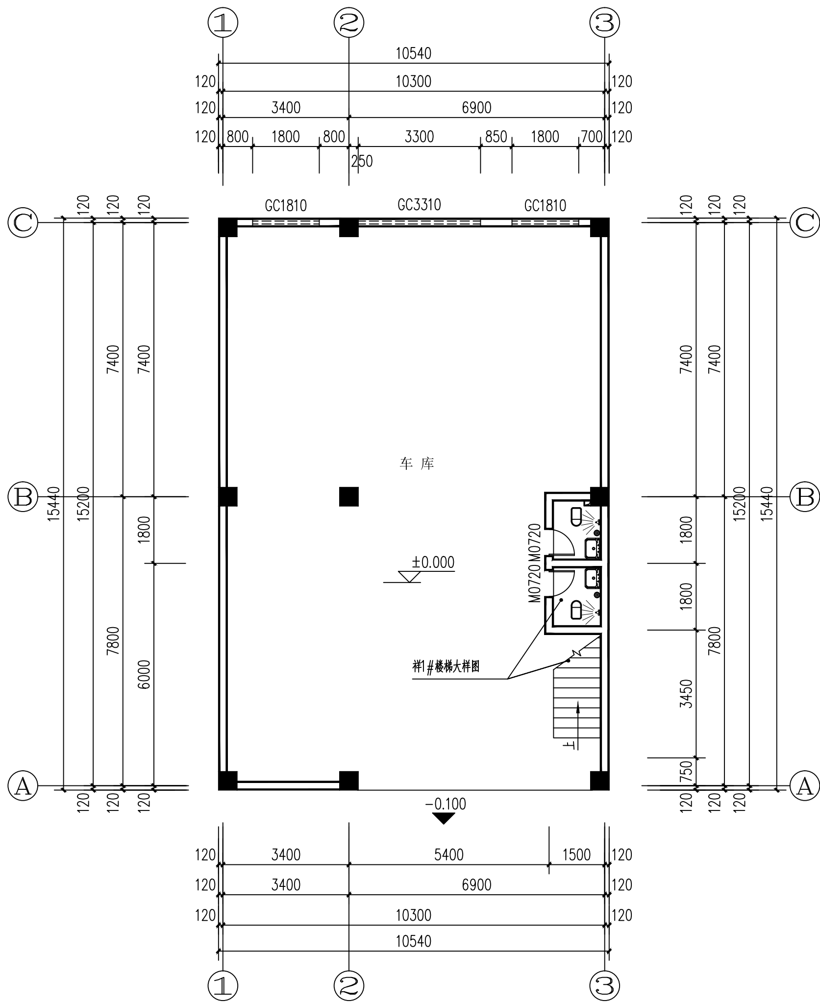
一层平面图
