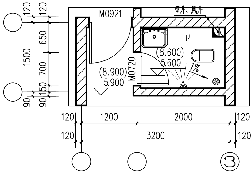
3#卫生间大样 1:50
