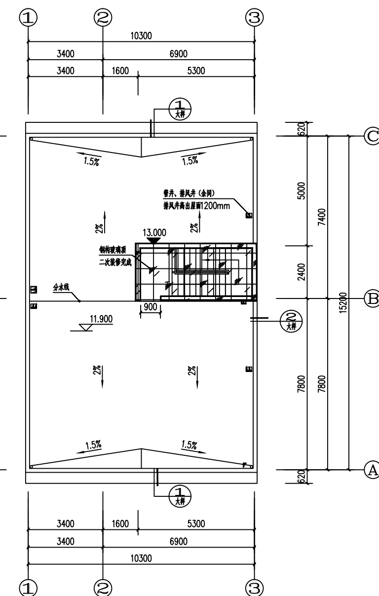
屋面平面图 1: 100
