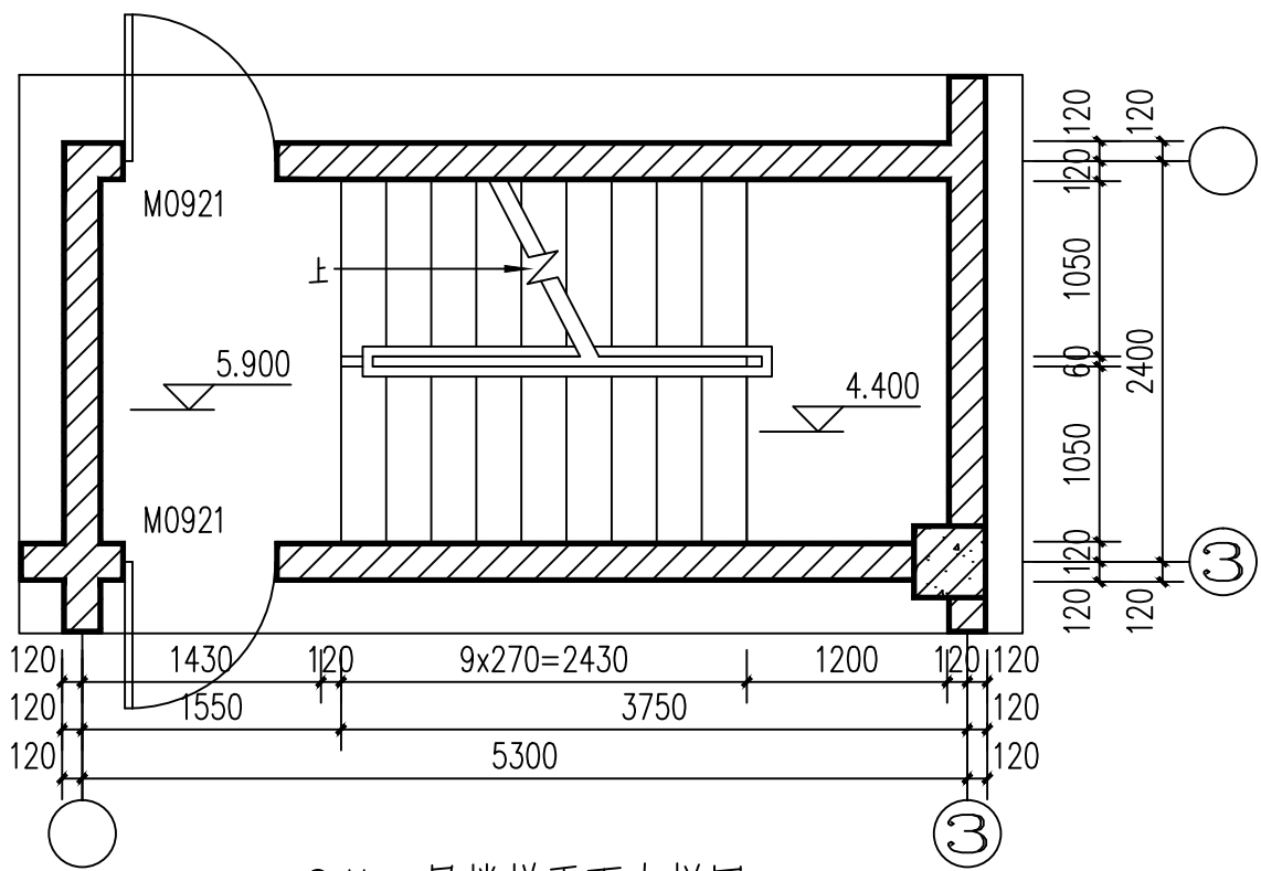
2#二层楼梯平面大样图 1:50
