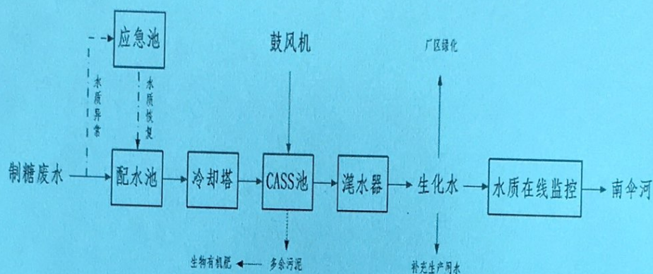
图 1 公司污水治理工艺流程图
